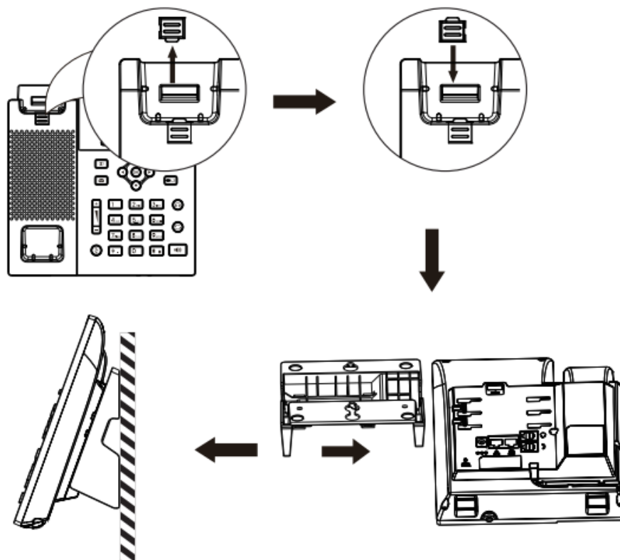
图 2 - 壁挂式安装
