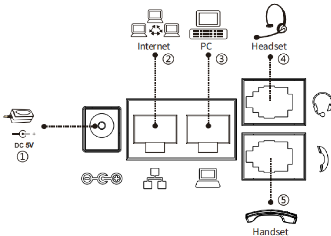
图 3 - 设备连接
