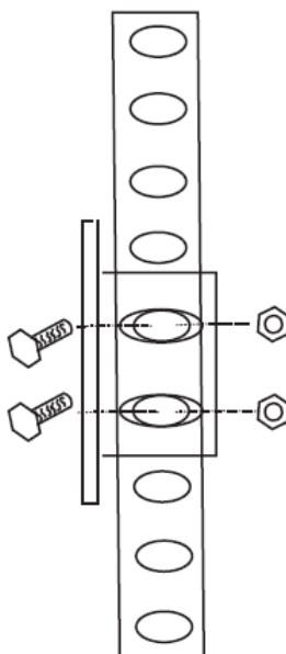
图 6：固定安装耳
