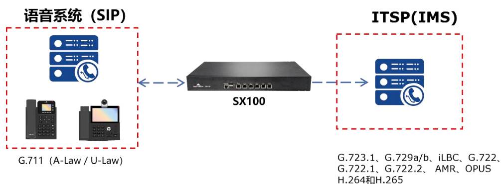
图 4: SX100 组网拓扑图
