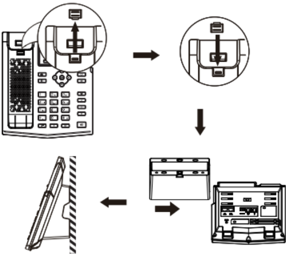
图 2 - 桌面式转化为壁挂式
