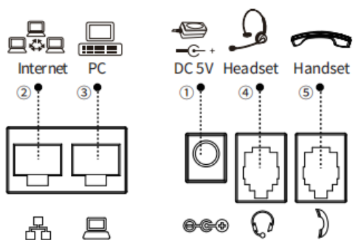
图 3 - 设备连接
