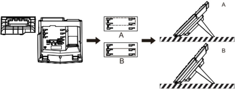
图 1- 桌面式话机安装
